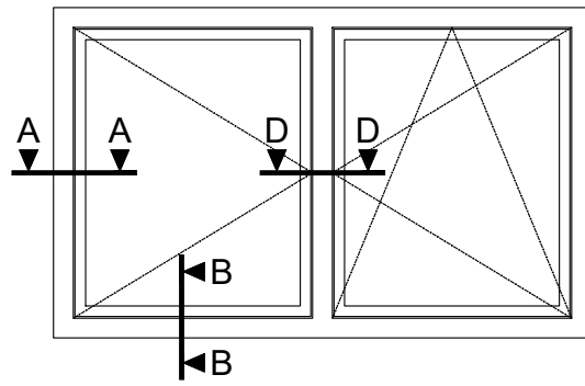
Zweiteilig mit Kämpfer Two-sash with mullion
