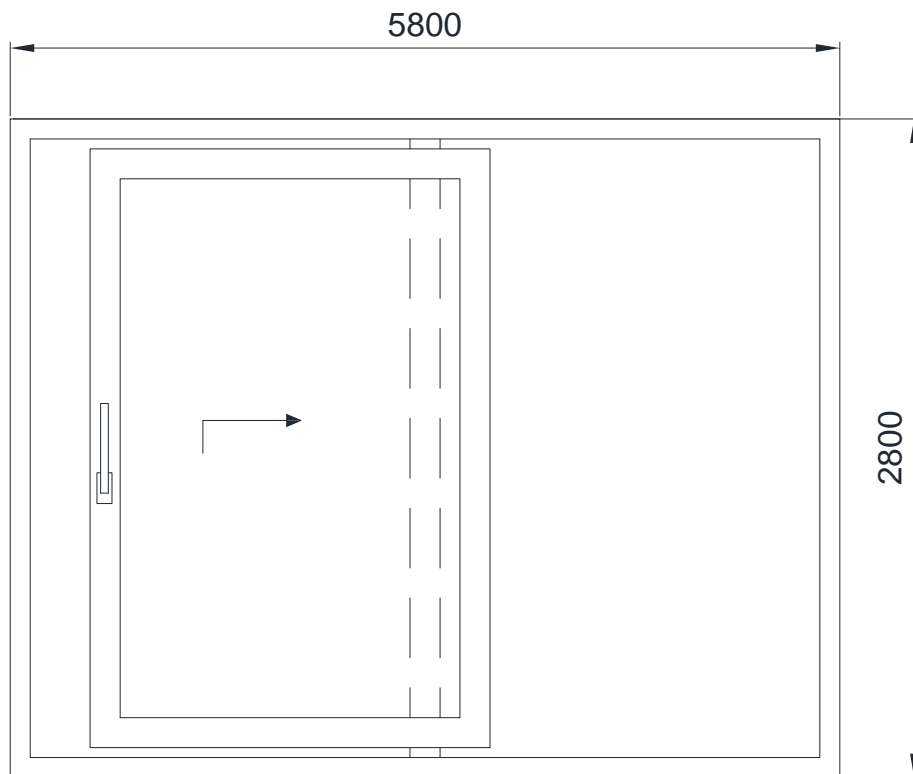
Bild 1: PK13, Ansicht Hebeschiebetüre (Darstellung nicht maßstabsgetreu)
