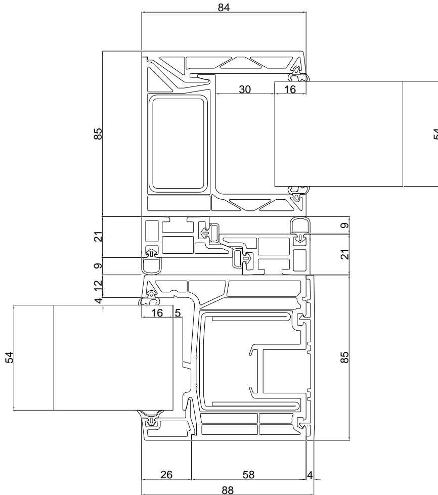
Bild 7: Profilquerschnitt PK06, Mittelschluss
