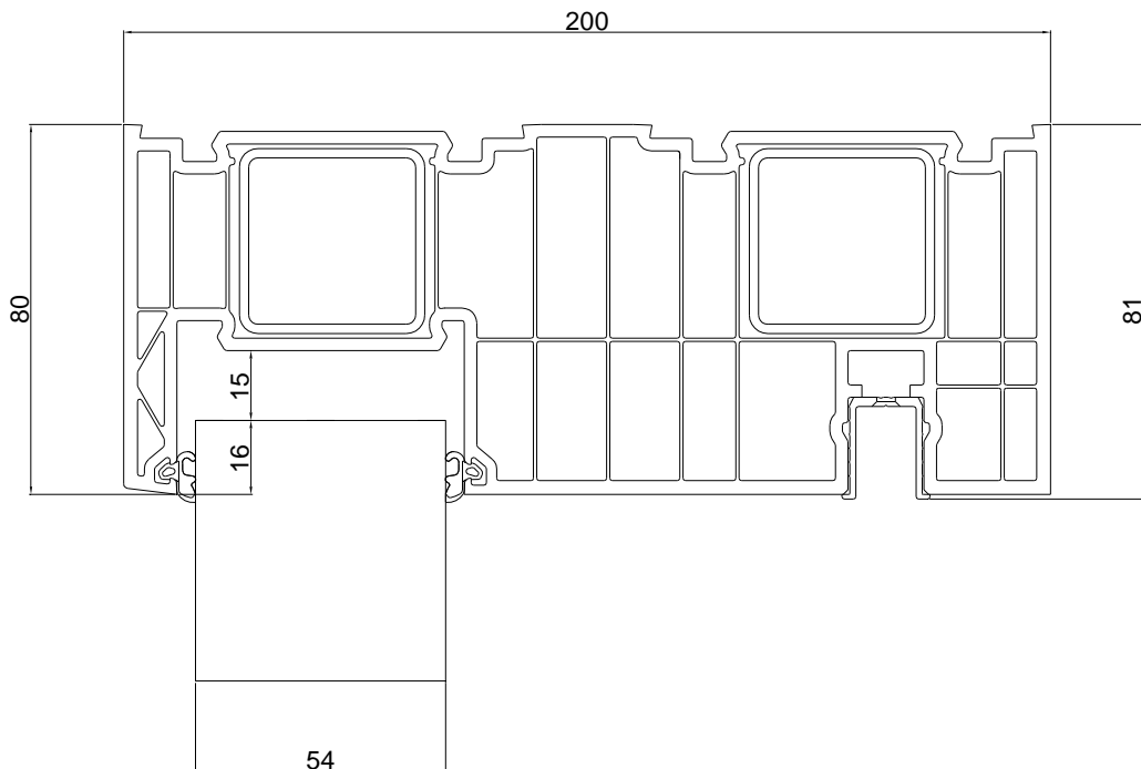
Bild 5: Profilquerschnitt PK04, Blendrahmen Standelement, oben und seitlich
