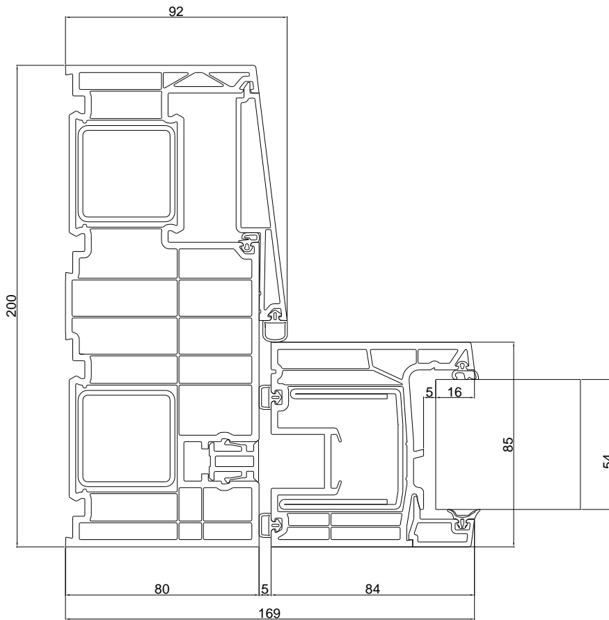
Bild 3: Profilquerschnitt PK02, Blendrahmen Schiebeelement, seitlich
