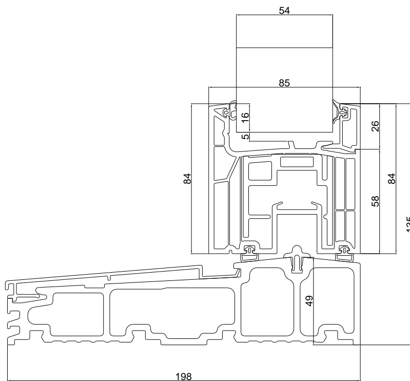
Bild 4: Profilquerschnitt PK03, Schwelle Schiebeelement
