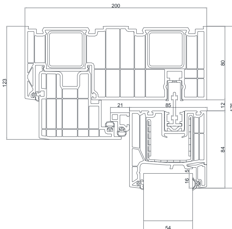
Bild 2: Profilquerschnitt PK01, Blendrahmen Schiebeelement, oben
