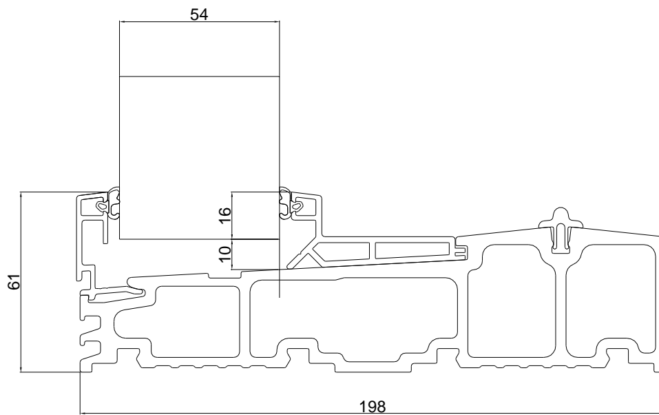
Bild 6: Profilquerschnitt PK05, Schwelle Standelement
